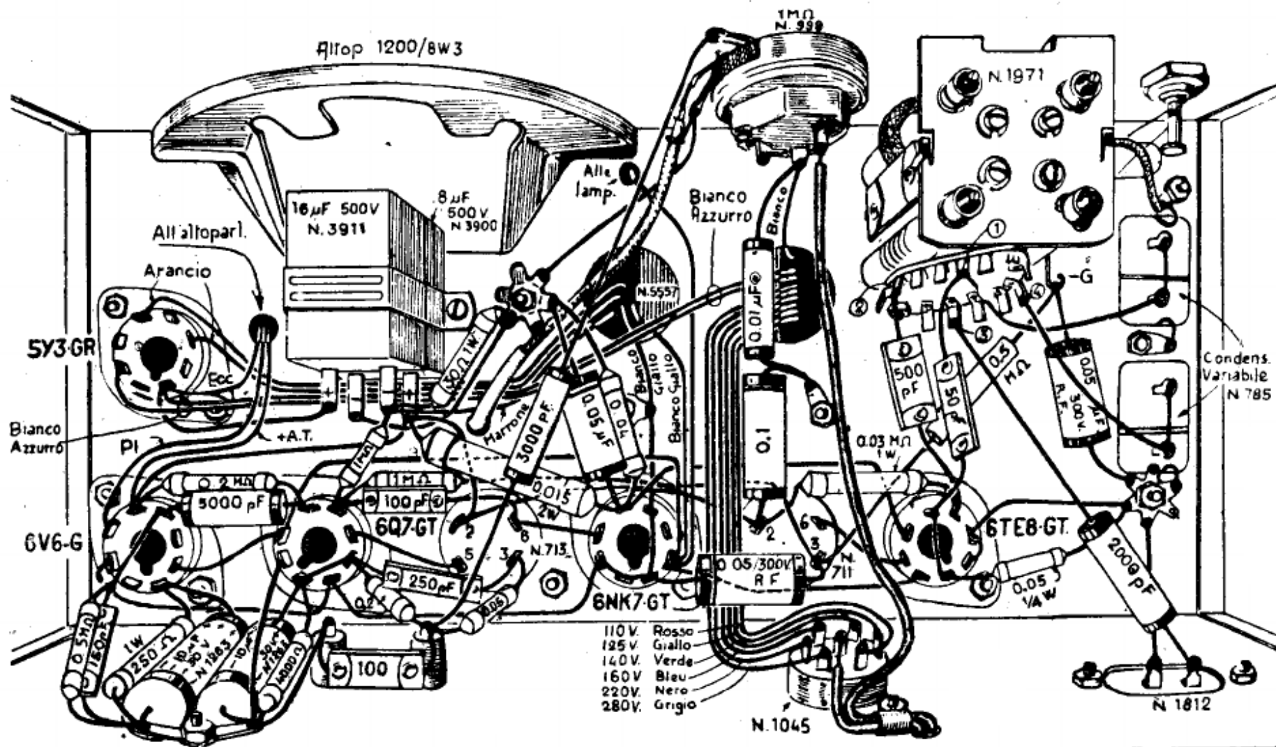
Lo schema costruttivo
